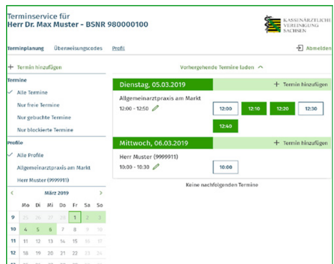
Gesamtansicht der Terminplanung mit Arztbezug
